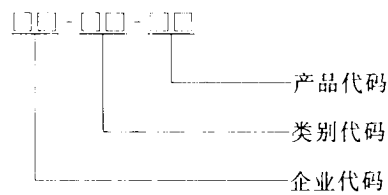
图 C.1 消防应急标志灯具的型号编制方法
